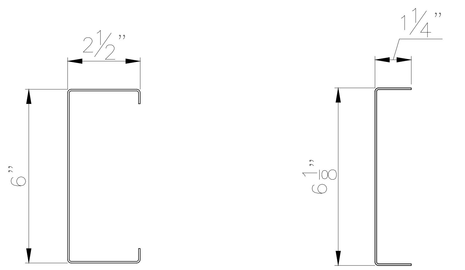
METAL STUD 16 GA. METAL TRACK 16 GA.
